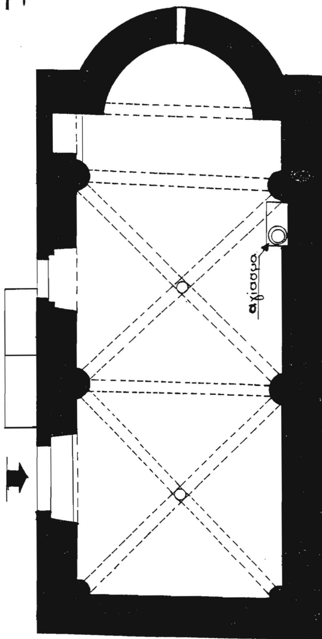
ΣΧΕΔ. 3 ΡΟΔΟΣ - ΜΑΣΑΡΙ - ΙΑΜΑΤΙΚΟ ΠΑΝΑΓΙΑ ΖΩΟΔΟΧΟΣ ΠΗΓΗ ΚΑΤΟΨΗ - ΚΛΙΜΑΚΑ 1:50
